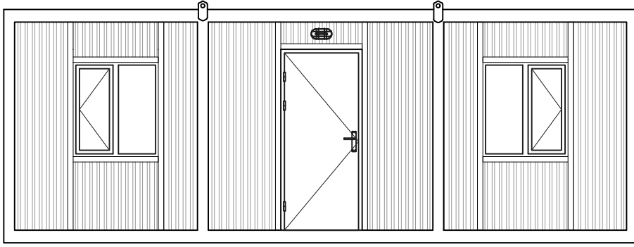
ÖN GÖRÜNÜŞ
