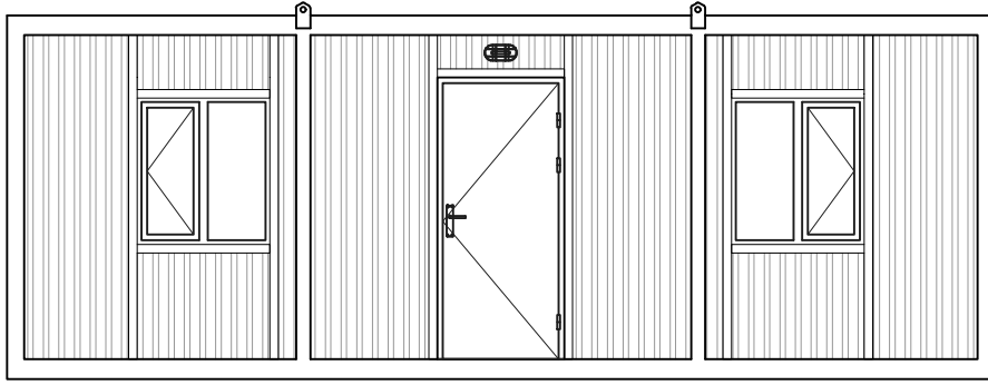
ÖN GÖRÜNÜS
