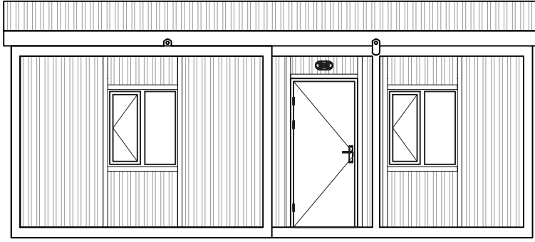
ÖN GÖRÜNÜS
